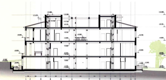
РАЗРЕЗ 2-2 М 1:150
