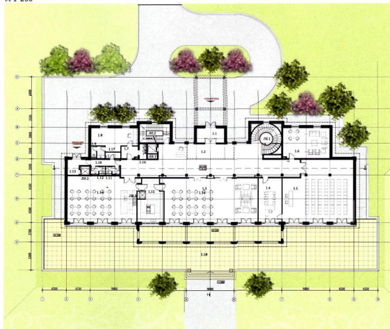
ПЛАН 1-ГО ЭТАЖА М 1-250
