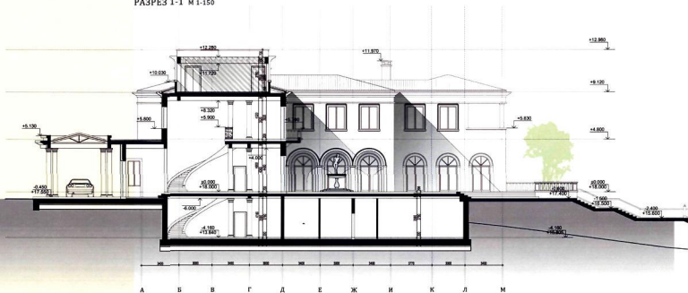
РАЗРЕЗ 1-1 М 1:150
