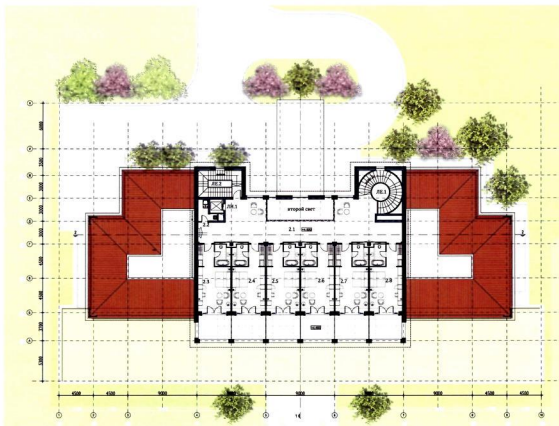
ПЛАН 2-ГО ЭТАЖА М 1-250
