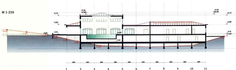
РАЗРЕЗ 2-2 М 1-250
